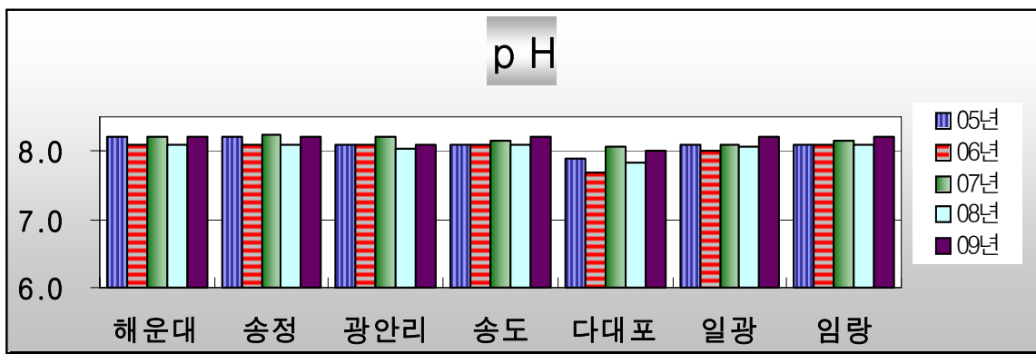
그림 1. 최근 5개년 간 해수욕장 pH 변화 추이
