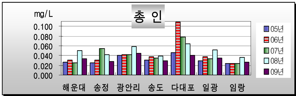
그림 4. 최근 5개년 간 해수욕장 총인 변화 추이
