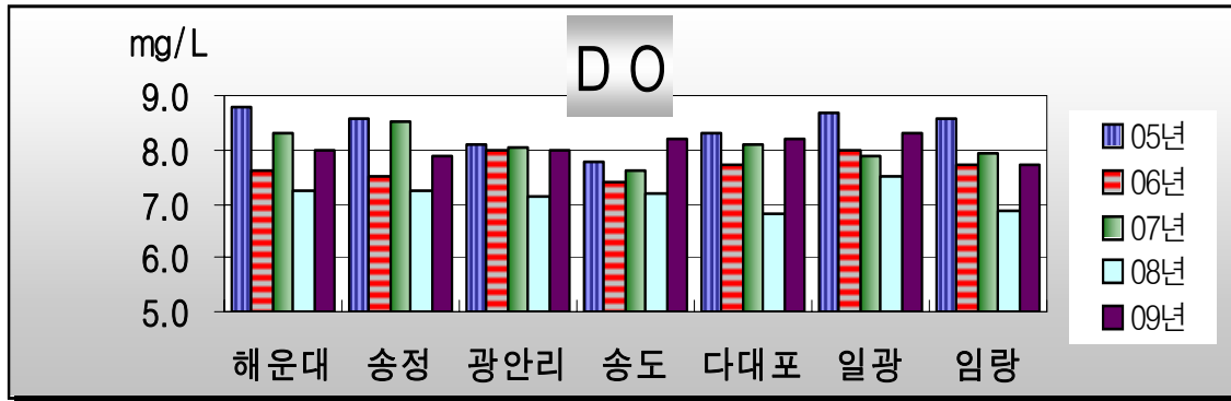
그림 2. 최근 5개년 간 해수욕장 DO변화 추이
