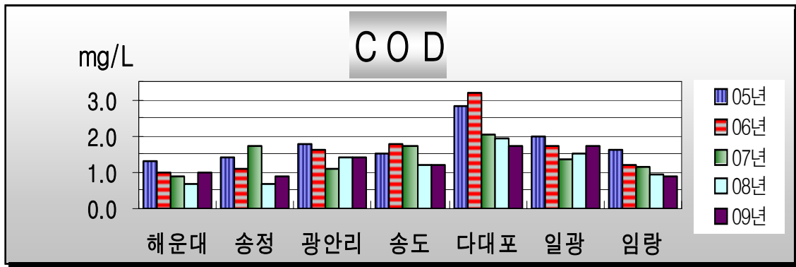
그림 3. 최근 5개년 간 해수욕장 COD변화 추이
