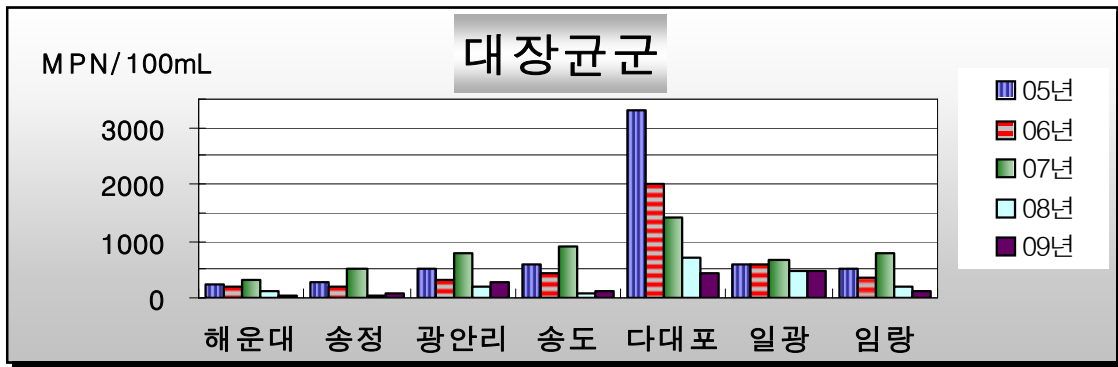
그림 5. 최근 5개년 간 해수욕장 대장균군 변화 추이
